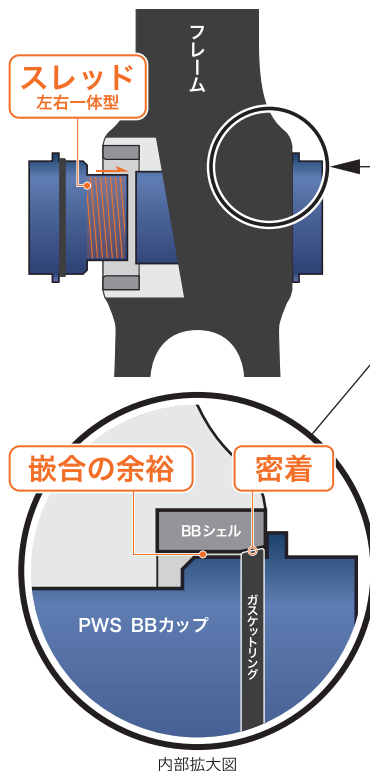
内部拡大図
